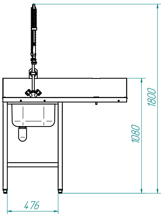
Левое исполнение
