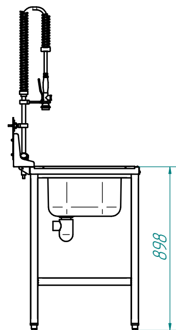
Правое исполнение
